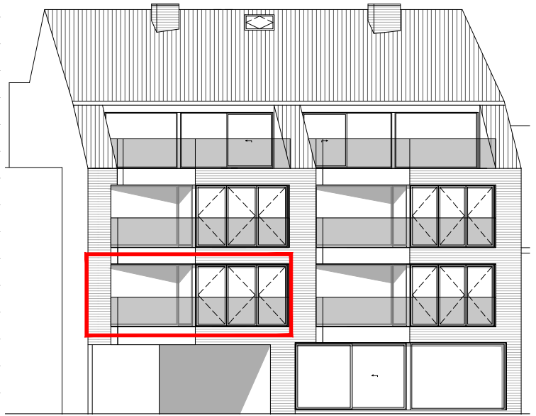
achtergevel - zuidoost
